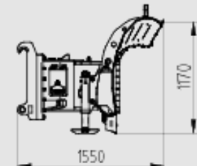
V-plow 3,2 m 1090 kg
