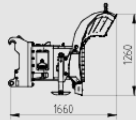
V-plow 3,7 m 1240 kg
